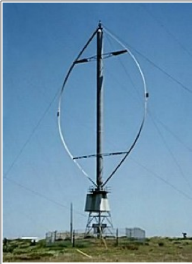
Éolienne de Darrieus
