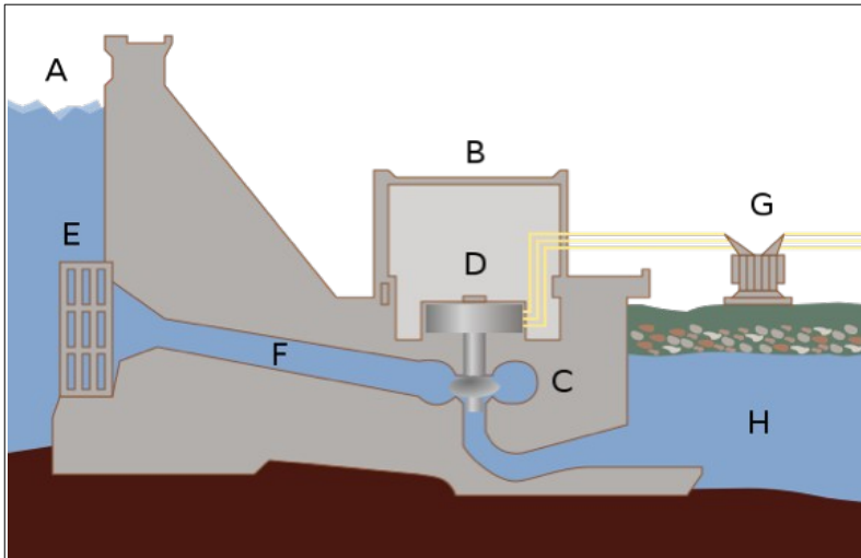
Schéma en coupe d'un barrage hydroélectrique.
