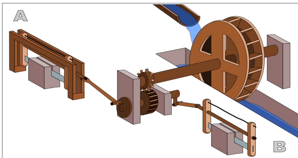
Scie hydraulique de Hiérapolis – IIIe siècle ap. J.C
