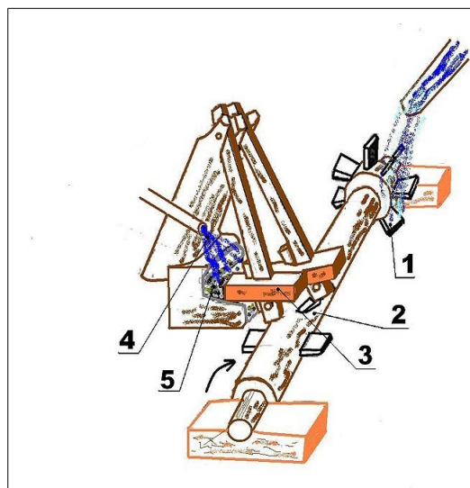
Schéma foulon: 1-roue à aubes, 2-arbres à cames, 3-maillets, 4-eau alcaline, 5-tissu à fouler
